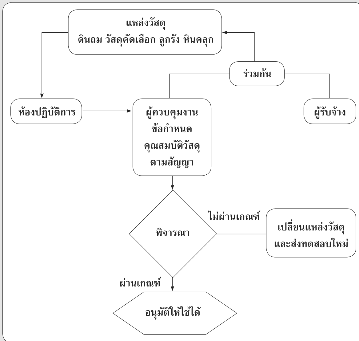
รูปที่ 3-2 ผังกระบวนการ General Test
