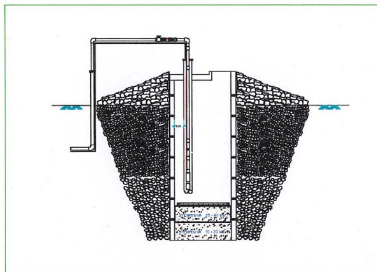
รูปที่ 35 เครื่องสูบน้ำคืบติดตั้งในถังกรองได้น้ำ
