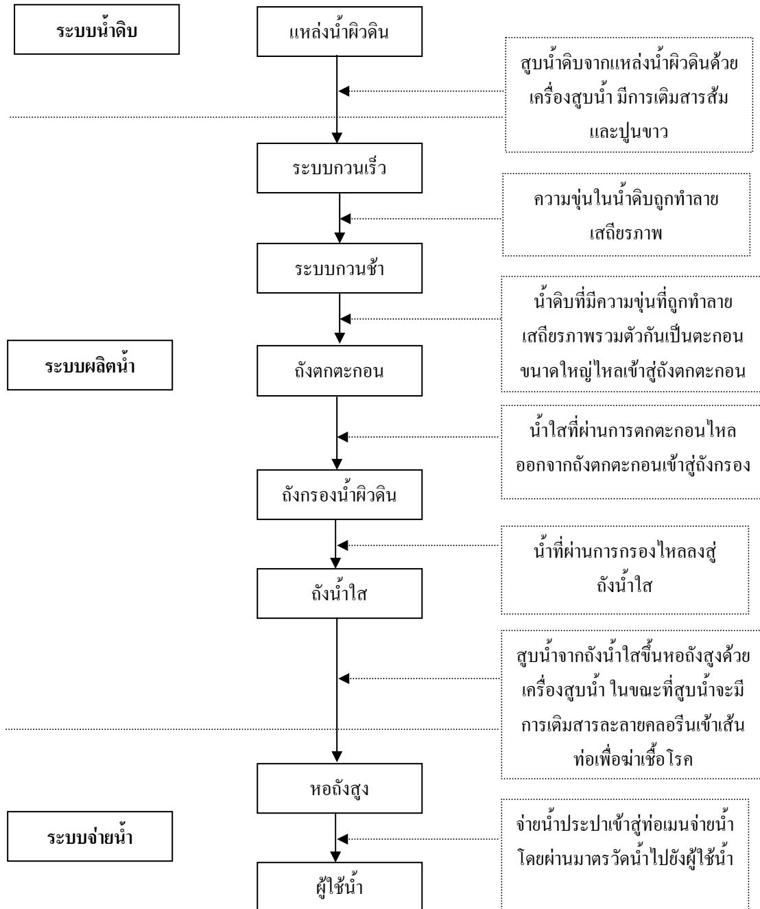
รูปที่ 14 สรุปกระบวนการผลิตน้ำประปาแบบผิวดิน
